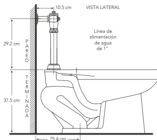
GRÁFICO REFERENCIAL DE INSTALACIÓN
